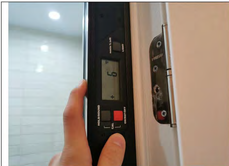
Фото №52. Отклонение коробки деревянного дверного блока от уровня вертикальности в ванной комнате.
