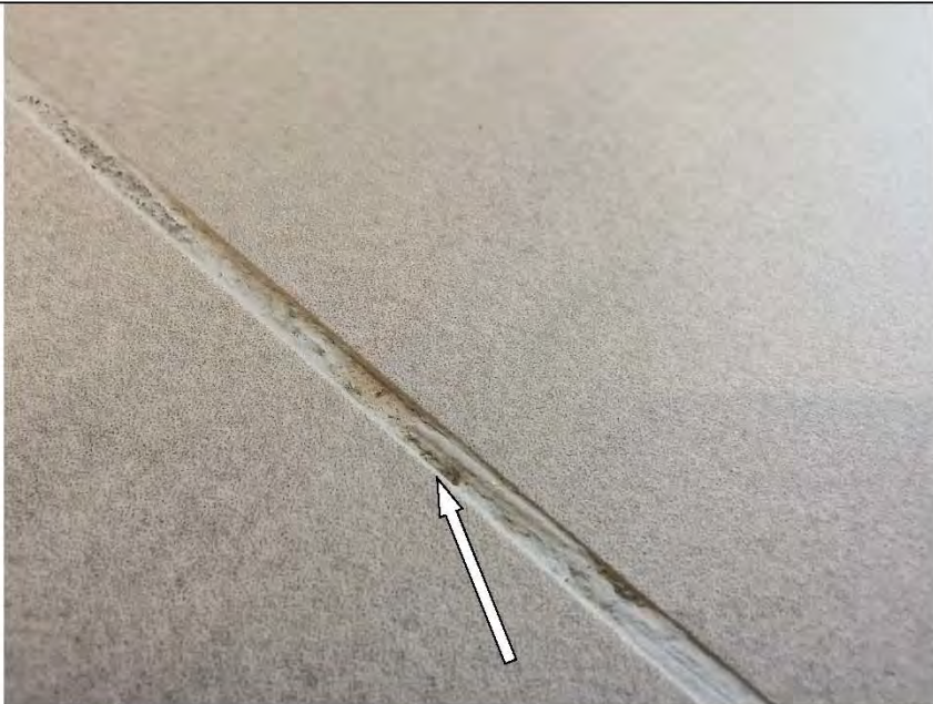
Фото №28. Неполное заполнение шовного пространства напольной керамической плитки затирочным составом в коридоре.
