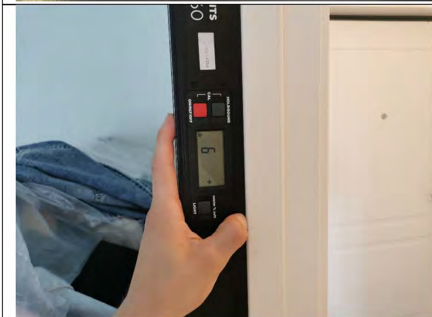
Фото №51. Отклонение коробки деревянного дверного блока от уровня вертикальности в спальне.
