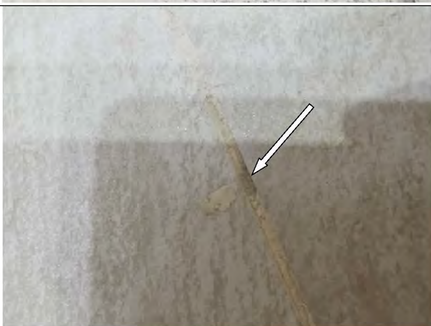
Фото №30. Неполное заполнение шовного пространства напольной керамической плитки затирочным составом на лоджии.
